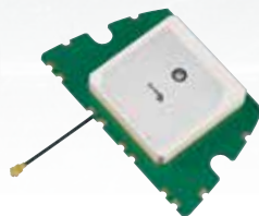
GPSGLONASS08N-S3-03-A 70x46x9 mm
