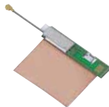
GPS396N-S3-00-A 37.0x8.0x2.5mm
